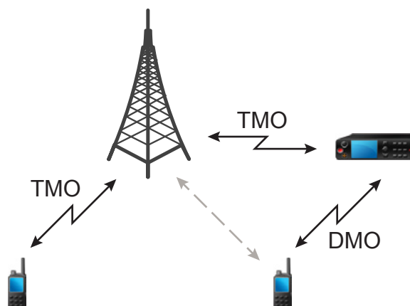
Abbildung 7: Gateway-Modus-Betrieb
